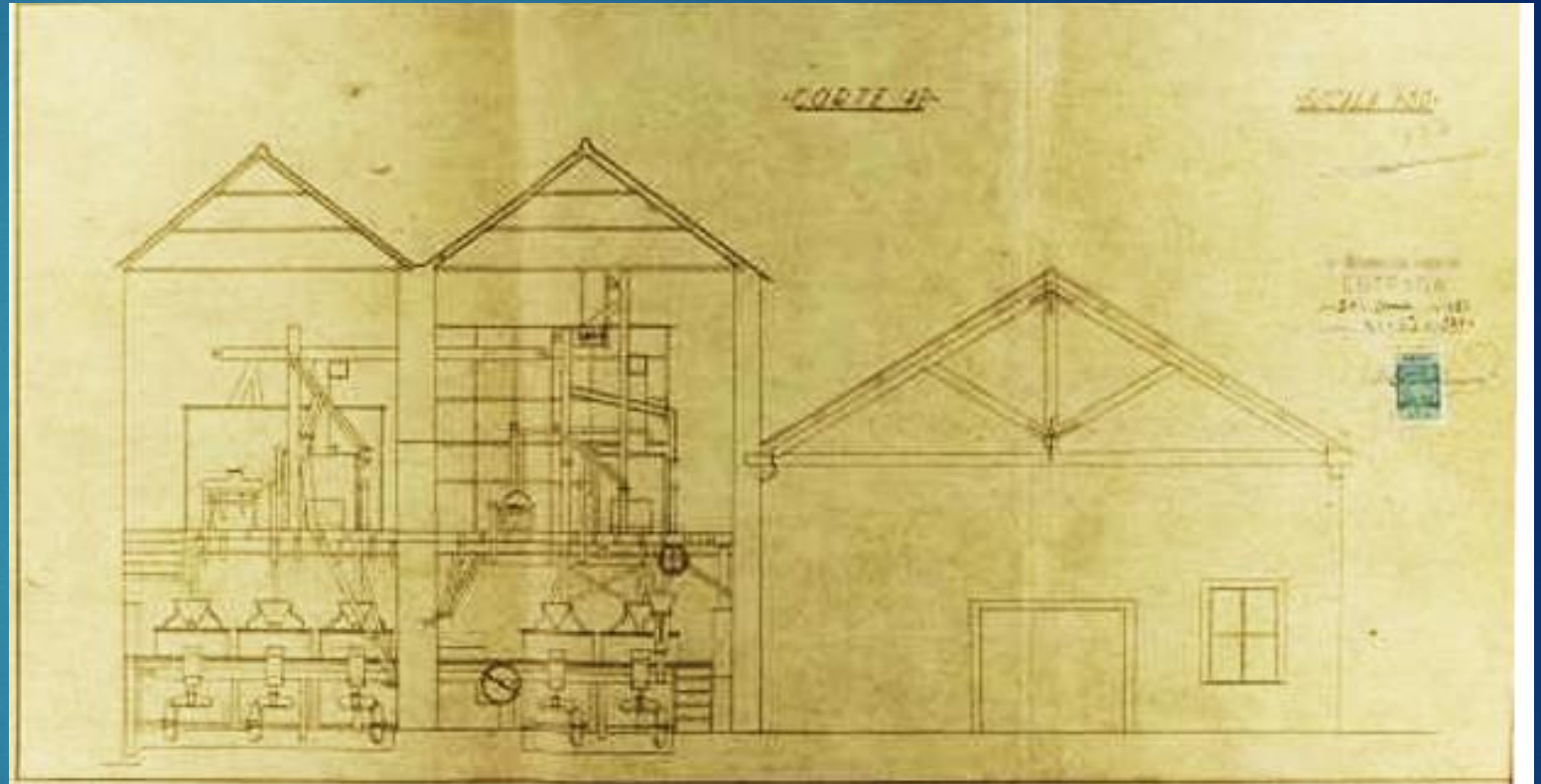
Figura 5 – Planta da moagem de Araújo Ribeiro & Dias, Lda., na Rua Jacques Pessoa, Tavira, já com a nova secção de moagem de milho e centeio (esquerda) acrescentada à anterior de trigo (direita), ca. 1942 Fonte: Arquivo Distrital de Faro, 5.ª Circunscrição Industrial (PT/ADFAR/ACD/C15/004-018/0012)
