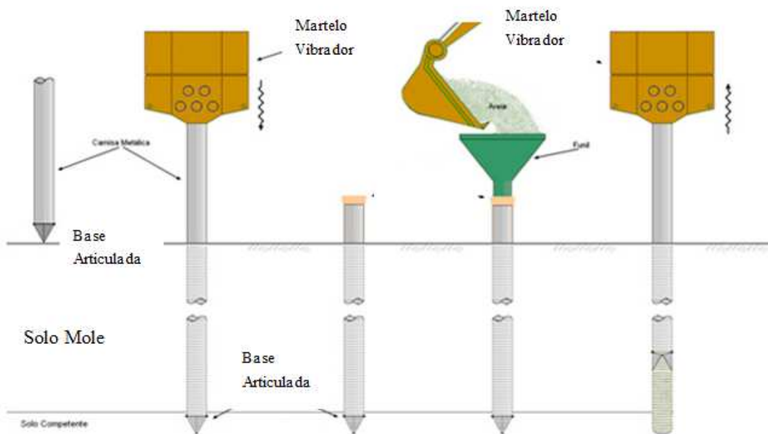
Fig.5 – Esquema de execução de um dreno de areia com recurso a Mandril Impulsionado (imagem retirada de http://www.stabtecn.com.br/servicos , em Abril de 2015)
