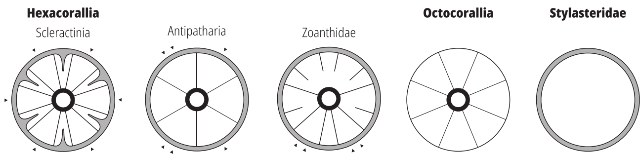
Figura 5. Diagrama da secção transversal dos pólipos dos principais taxa de corais, ilustrando as maiores diferenças. A área sombreada indica o exosqueleto; o círculo central representa a boca e a actino-faringe; as linhas radiais indicam os mesentérios: completos (ou perfeitos) quando atingem a actino-faringe e incompletos (ou imperfeitos) quando tal não acontece. As setas indicam regiões onde se formam mesentérios adicionais após os primeiros 6 ou 12. (Adaptado de Roberts et al. , 2009)
