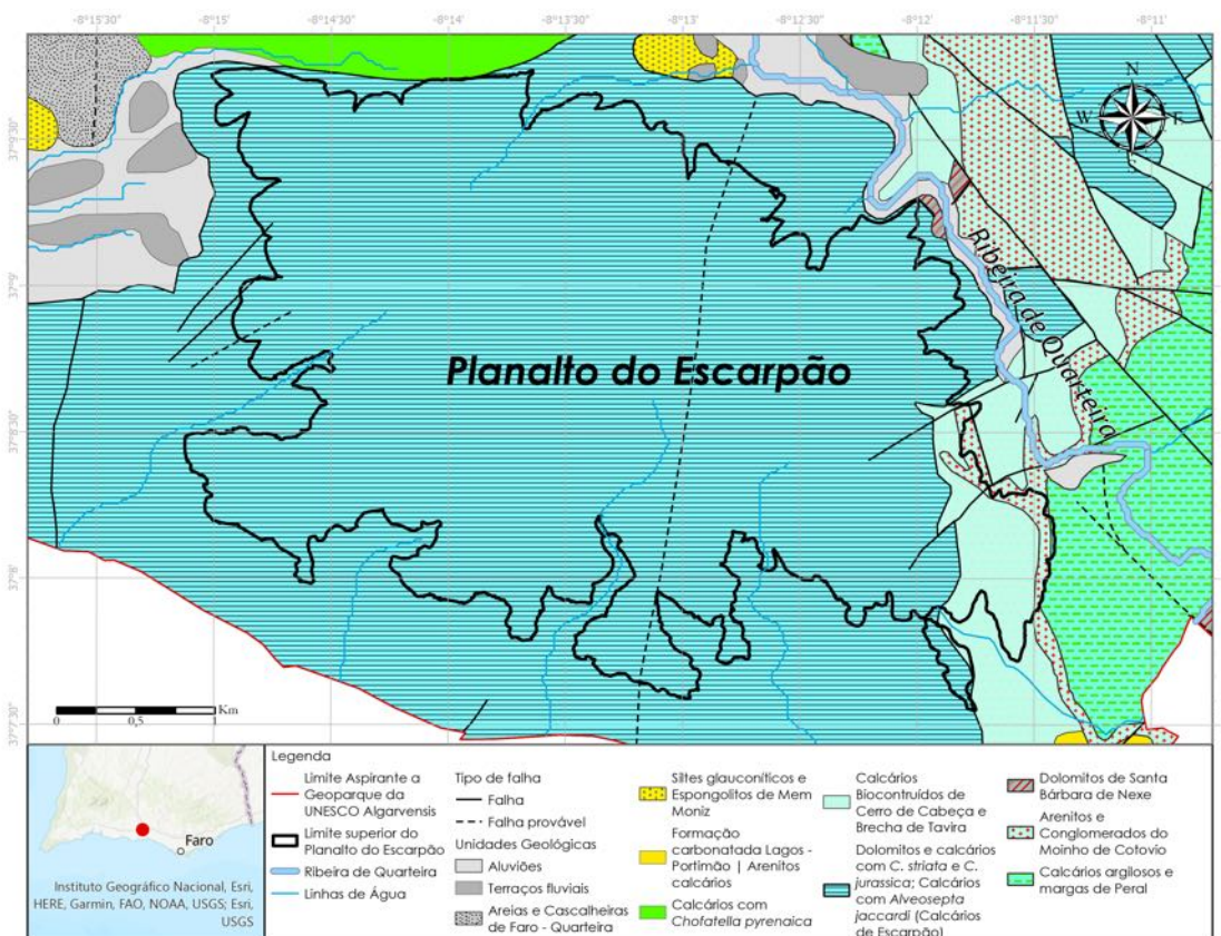
Figura 4.1. Localização e geologia do Planalto do Escarpão.
