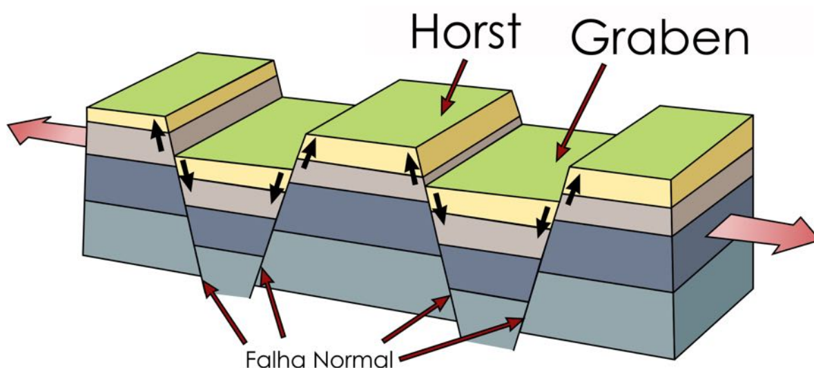
Figura 5.2. Estruturas geológicas em horst-graben.
