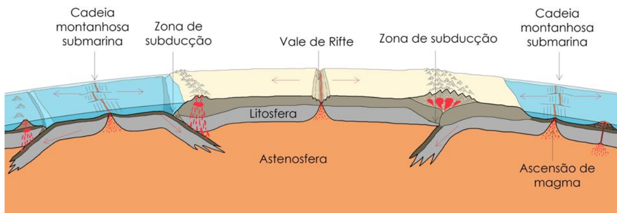
Figura 2.3. Esquema dos processos envolvidos na deriva continental- tectônica de placas. A litosfera é a camada sólida mais exterior da Terra, com espessura variável, sendo mais espessa por baixo das cadeias montanhosas; a astenosfera é a zona do manto terrestre, menos rígida que a litosfera, que se situa entre aproximadamente 80 e 200 km abaixo da superfície.
