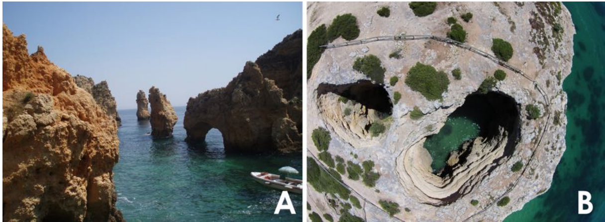
Figura 7.4. A: Ponta da Piedade, Lagos (Algarve); B: imagem drone dos algarves de Albandeira, Algarve
