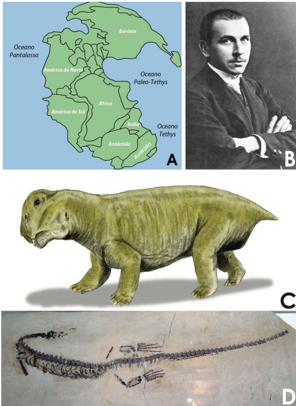
Figura 2.2. A: supercontinente Pangeia na Era Paleozoica, entre 541-252 milhões de anos (ver Figura 1.1). O oceano que rodeava a Pangeia designa-se por Panthalassa; B: retrato de Alfred Wegener (autor desconhecido, 1910); C: desenho de Lystrosaurus murrayi do início do Triássico (ca. 250 milhões de anos), encontrado na África do Sul; D: Mesosaurus (réptil aquático da Era Paleozoica), cujos fósseis se encontram em ambos os continentes América do Sul e África.
