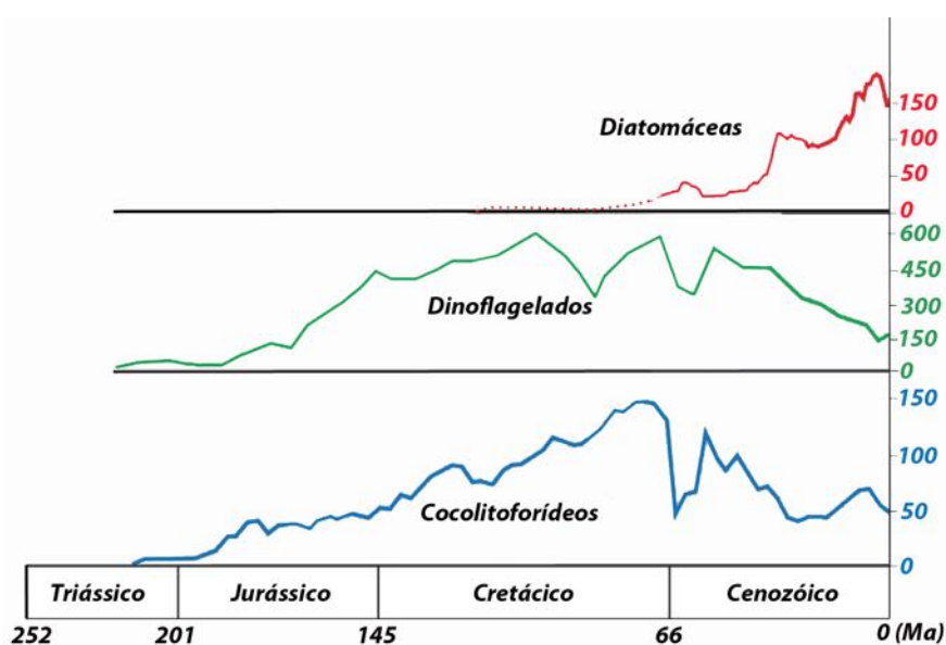
Figura 3.13. Evolução do número de espécies fitoplanctônicas durante o Mesozoico e o Cenozoico (ver tabela cronostatigráfica da Figura 1.1). No eixo horizontal, Ma= milhões de anos. No eixo vertical: número de espécies.
