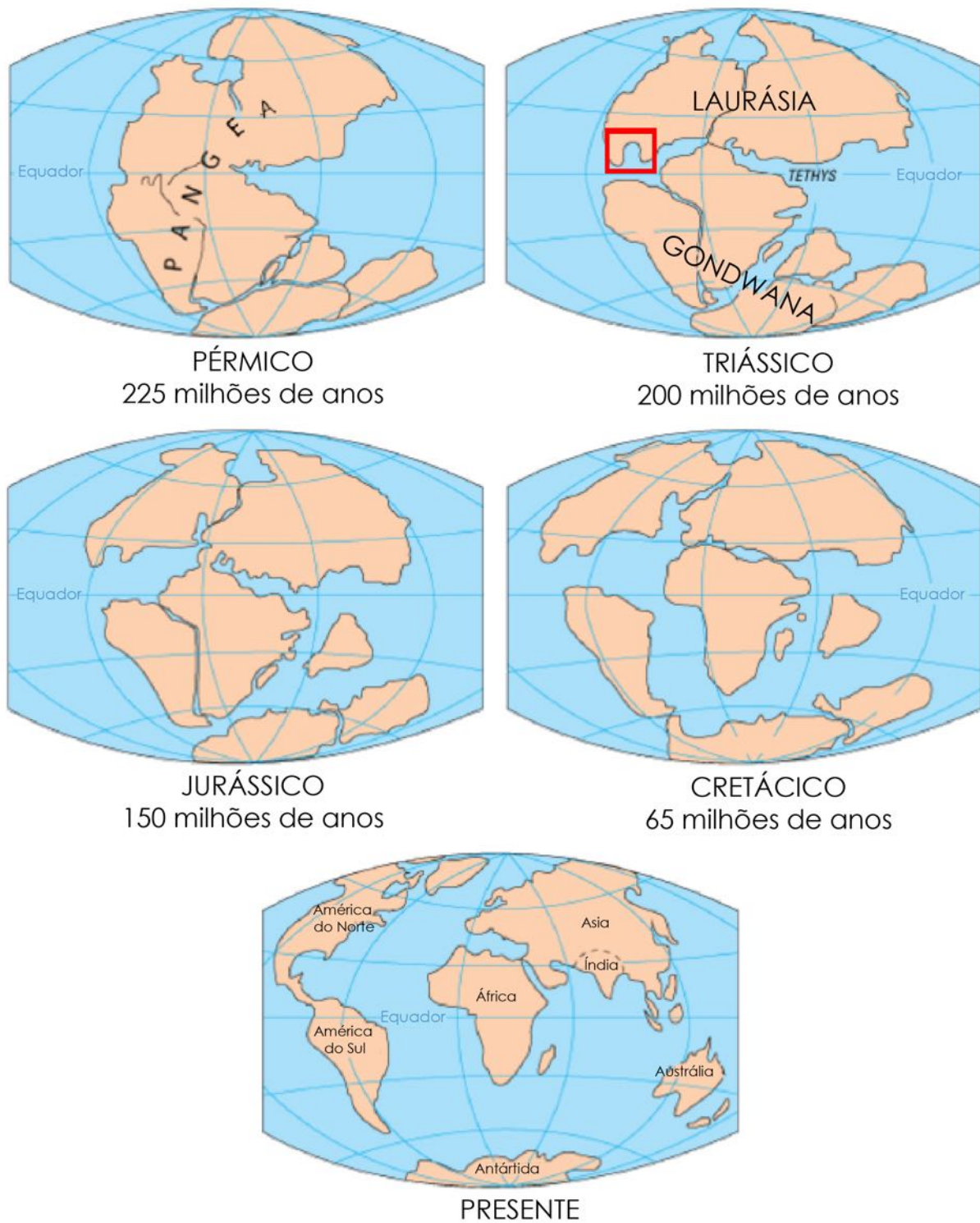
Figura 2.6. Evolução paleogeográfica dos continentes entre os 225 milhões de anos e o atual. O quadrado vermelho, indica a posição do Golfo do México no Triássico.
