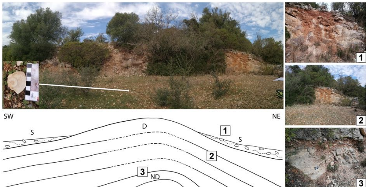
Figura 6.5. Cerro Monchina. Em cima: fotografia de dobra em anticlinal nos Calcários e Margas de Telheiro e fósil de amonite encontrado no solo; Em baixo: esquema interpretativo do corte geológico na vertente sul do Cerro Monchina, correspondente à fotografia A, em que 1) pormenor das camadas no flanco nordeste da dobra e solo (s); 2) camadas de espessura métrica, inclinando 60° para este; 3) núcleo da dobra (ND). As linhas a tracejado no esquema B, correspondem à massa de rocha que desapareceu por erosão.
