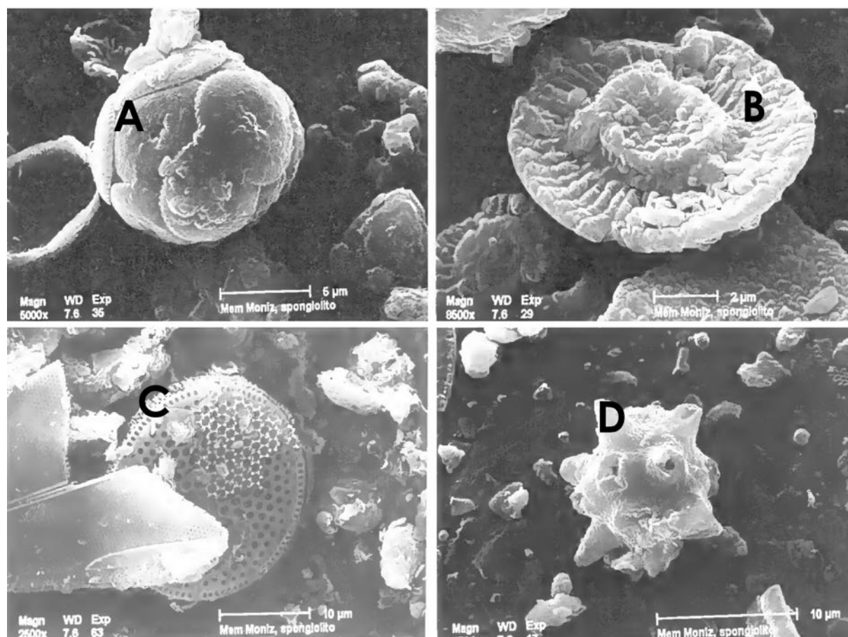
Figura 5.9. Microfósseis dos Espongólitos de Mem Moniz. A: Reticulofenestra minuta (coccosfera); B: Coccolithus miopelagicus (coccosfera); C: Coscinodiscus tuberculatus (diatomácea); D: Microscleva (esponja). Nota: 1µm=0,01 milímetros.
