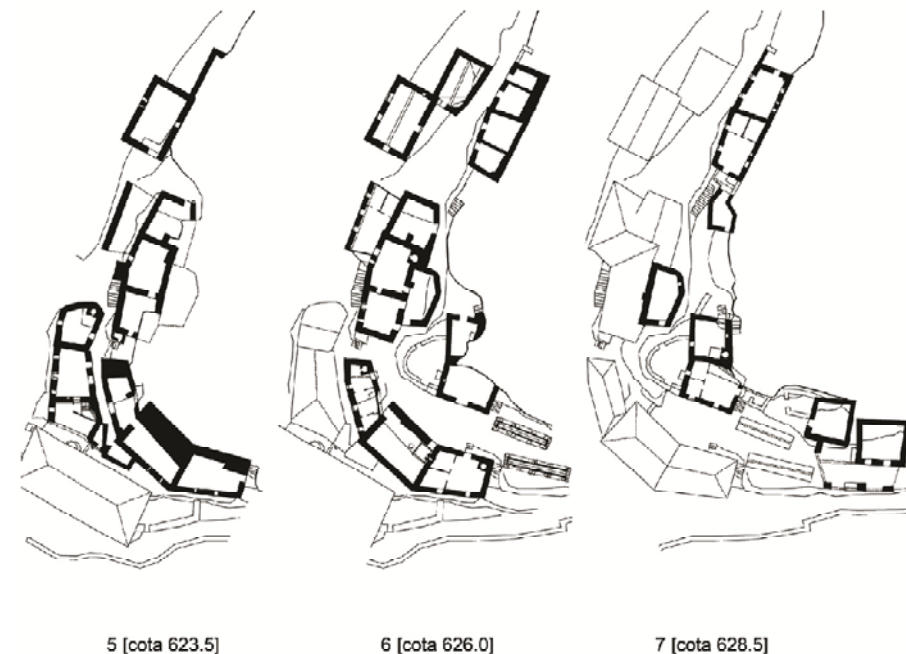
Fig. 1 Planta parcial do lugar da Drave (sete cotas diferenciadas), escala 1/1000 (mrc)
