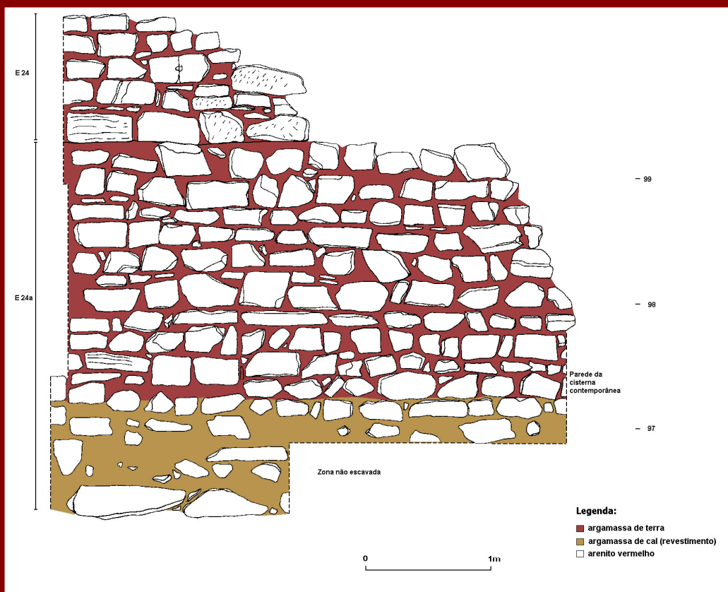
Fig. 20 - Estrutura 24 - Muro de contenção (?)
