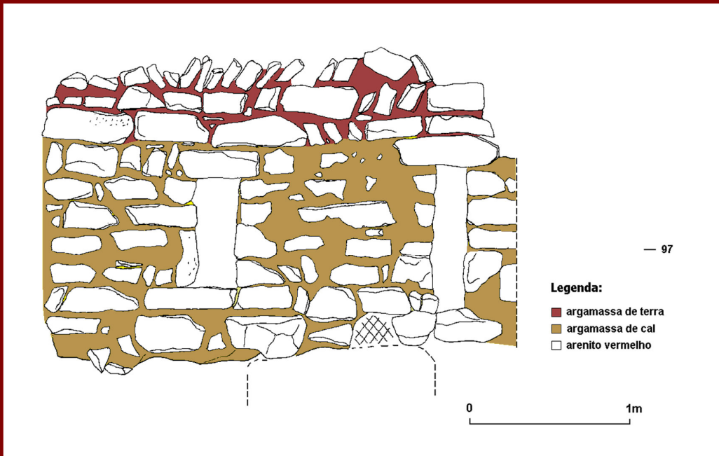
Fig. 21 - Muro de contenção e drenagem (estrutura 46/46A)
