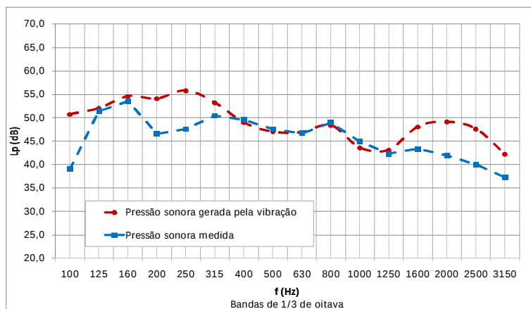
Figura 6: Níveis Sonoros previstos (vibração) e medidos
