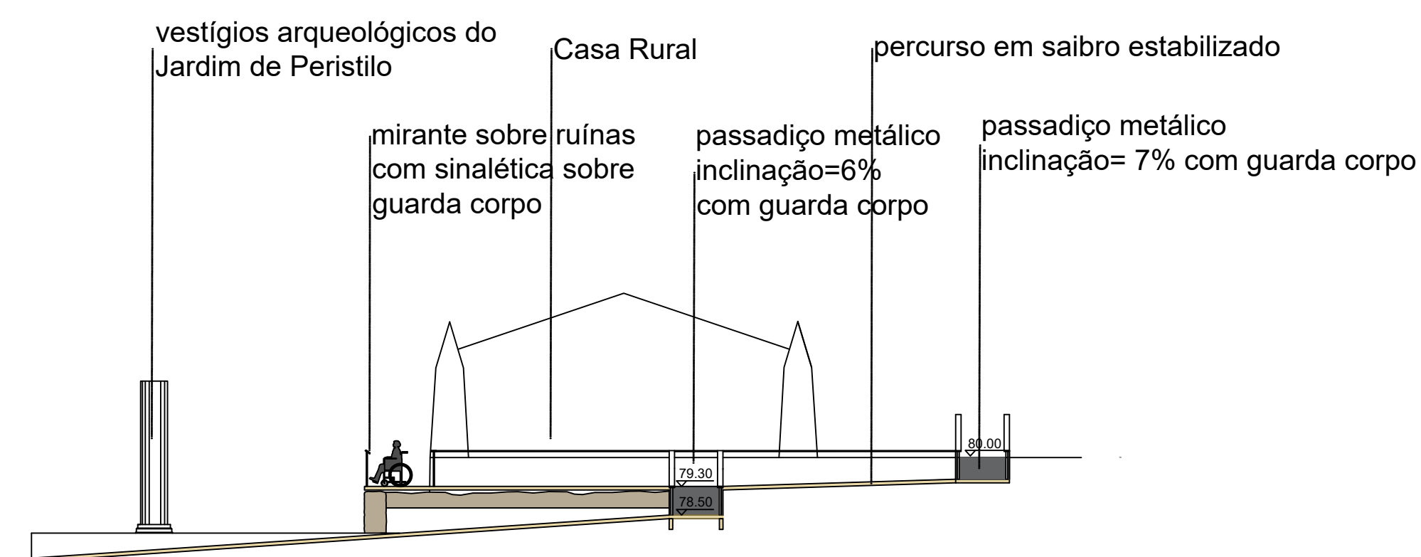
corte CC
