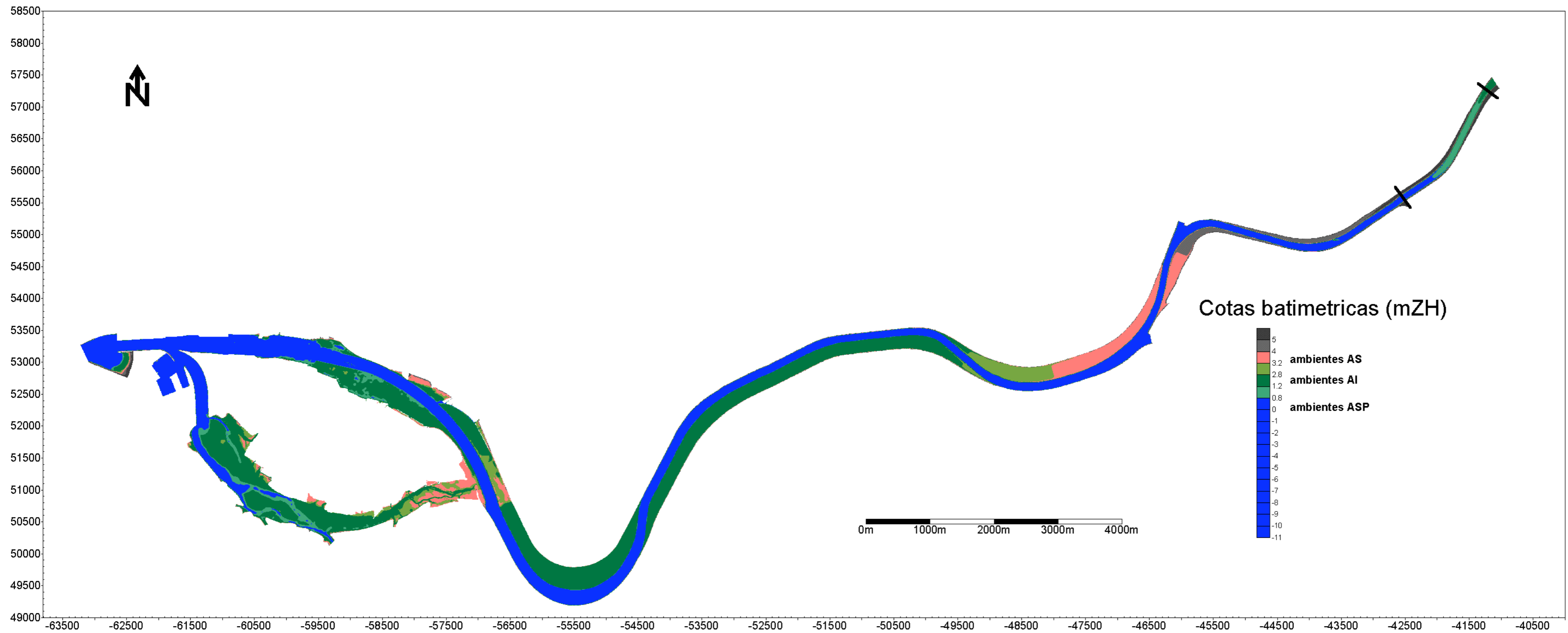
Figura 5.2.2. Distribuição espacial dos diferentes ambientes definidos pela variação da superfície livre no estuário do Mondego, em 1995 durante os trabalhos de regularização do braço norte. Para os ambientes localizados abaixo do patamar médio h_{xy} < +0.8\text{mZH} foram definidos os ambientes permanentemente imersos (ASP), para as zonas compreendidas entre os +0.8 \leq h_{xy} < +1.2\text{mZH} foram cartografados os ambientes esporadicamente emersos apenas durante as marés vivas (AIEI). Os ambientes intermareais mais frequentes (AIF) foram definidos para +1.2 \leq h_{xy} \leq +2.8\text{mZH} , enquanto os ambientes esporadicamente imersos apenas durante as marés vivas (AIES) para +2.8 < h_{xy} \leq +3.2\text{mZH} . Os locais do estuário inundados apenas durante quadros de marés de maior amplitude associados ou a sobre-elevação do nível do mar por fenómeno atmosféricos e/ou a grandes cheias do Mondego (AS), foram definidos para níveis compreendidos entre +3.2 < h_{xy} \leq +4.0\text{mZH} .
