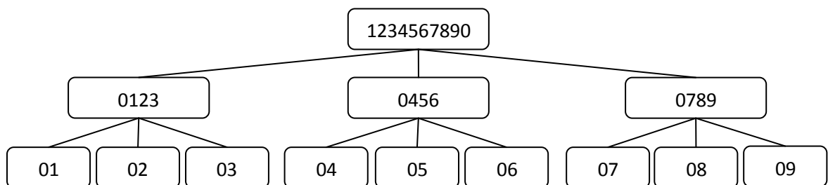
Figura 4.1.y - Representação da organização hierárquica dos números.
