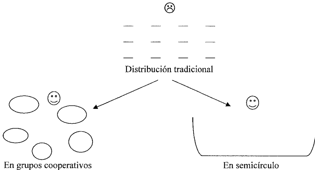
Esquema 3
