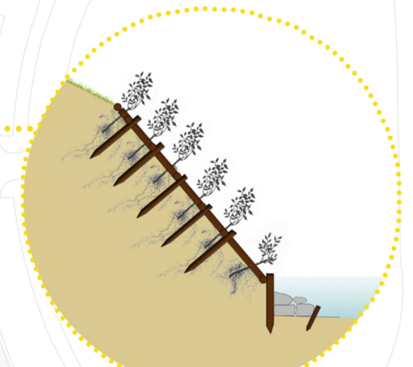
Solução tipo - Grade viva. S/ Escala
