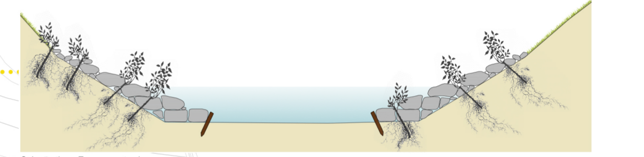
Solução tipo - Enrocamento vivo. Escala 1:50
