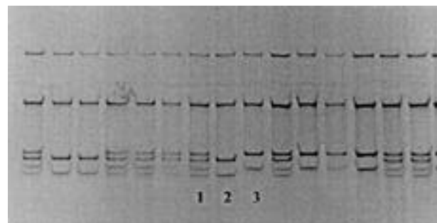
Figure 2. SSCP analysis of the 166bp fragment of \alpha -La gene. Electrophoresis was performed in a 14% acrylamide gel, without glycerol, at 400 V and 15 °C for 7 h, using 10 \mu l of DNA and 15 \mu l of denaturing solution. The frequencies of the three conformational patterns detected were 57.5% for pattern 1, 22.5% for pattern 2 and 20% for pattern 3— Analyse SSCP du fragment de 166 pb du gene de \alpha -La. L'électrophorèse a été réalisée sur un gel de polyacrylamide à 14 %, sans glycérol, à 400 V et à 15 °C pendant 7 h, utilisant 10 \mu l de DNA et 15 \mu l de solution dénaturante. Les fréquences des trois profils conformationnels détectés ont été 57,5 % pour le profil 1, 22,5 % pour le profil 2 et 20 % pour le profil 3.
