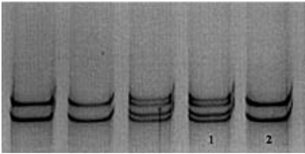
Figure 3. SSCP analysis of the 510bp fragment of \beta -Cn gene. Five \mu l of amplified DNA and 15 \mu l of denaturing solution were run in a 15% acrylamide gel without glycerol. Electrophoresis was performed at 400 V and 15 °C for 16 h. The frequencies of the two conformational patterns detected were 37.5% for pattern 1 and 52.5% for pattern 2 — Analyse SSCP du fragment de 510 pb du gène de \beta -Cn. Cinq \mu l d'ADN amplifié et 15 \mu l d'une solution dénaturante ont été placés sur un gel de polyacrylamide à 15 % sans glycérol. L'électrophorèse a été réalisée à 400 V, à 15 °C pendant 16 h. Les fréquences des deux profils conformationnels détectés ont été de 37,5 % pour le profil 1 et de 52,5 % pour le profil 2.
