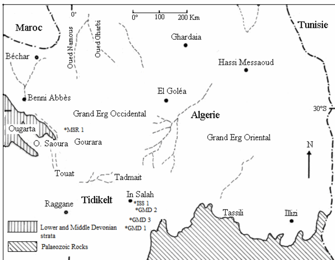
Figure 1. Carte général et de localisation des forages étudié.
