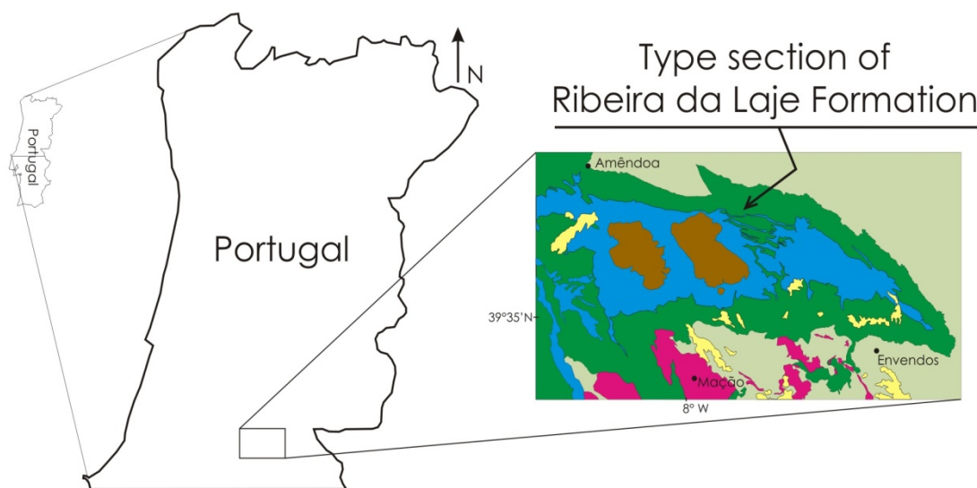
Figure 1. Localization of the Amêndoa/Mação Syncline and the type section of the Ribeira da Laje Formation (Adapted from: Geological Map of Portugal, 1/50 000 (28-A Mação), IGM, 2000).
