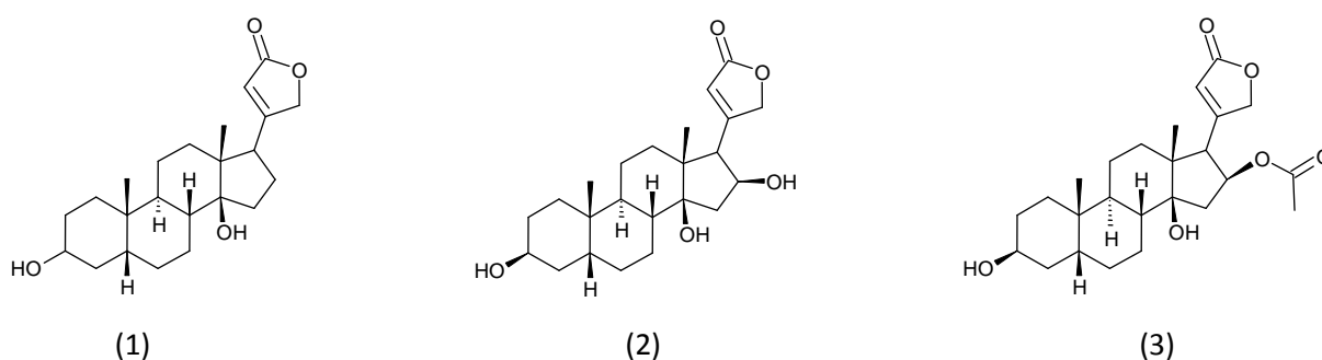
Figura 3.2: Estruturas de digitoxigenina (1), gitoxigenina (2) e gitaloxigenina (3).
