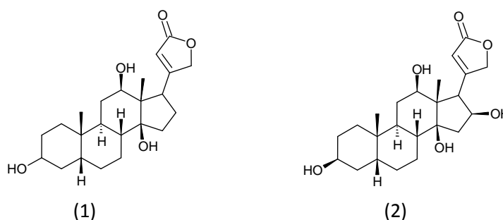
Figura 3.3: Estruturas de digoxigenina (1) e diginatinin (2).
