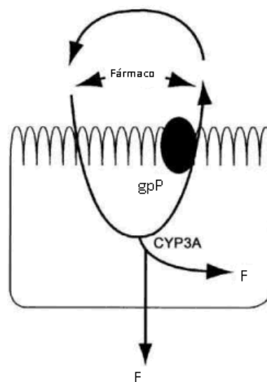
Figura 4.1: Glicoproteína-P na absorção intestinal dos fármacos (adaptado de http://www.farmacovigilanza.org/corsi/de_sarro3/corso2_frame.htm )
