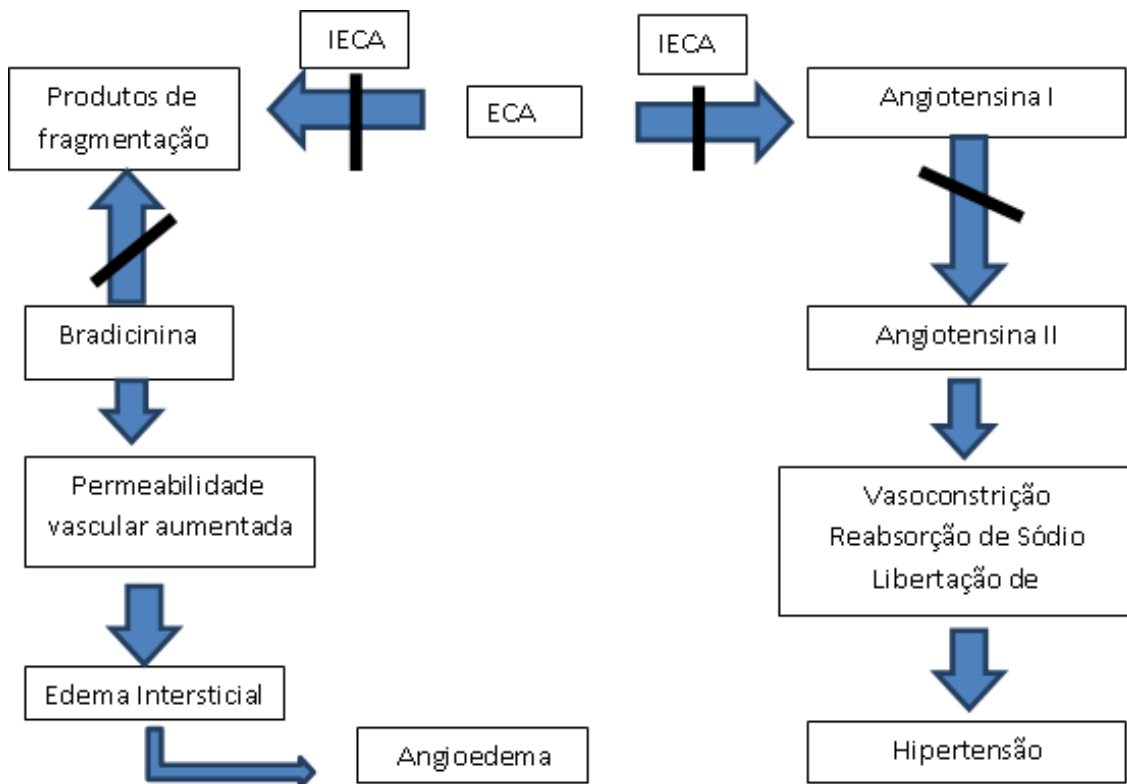
Figura 2.2: Mecanismo de Ação dos IECAs (adaptado do site Medscape 25 )
