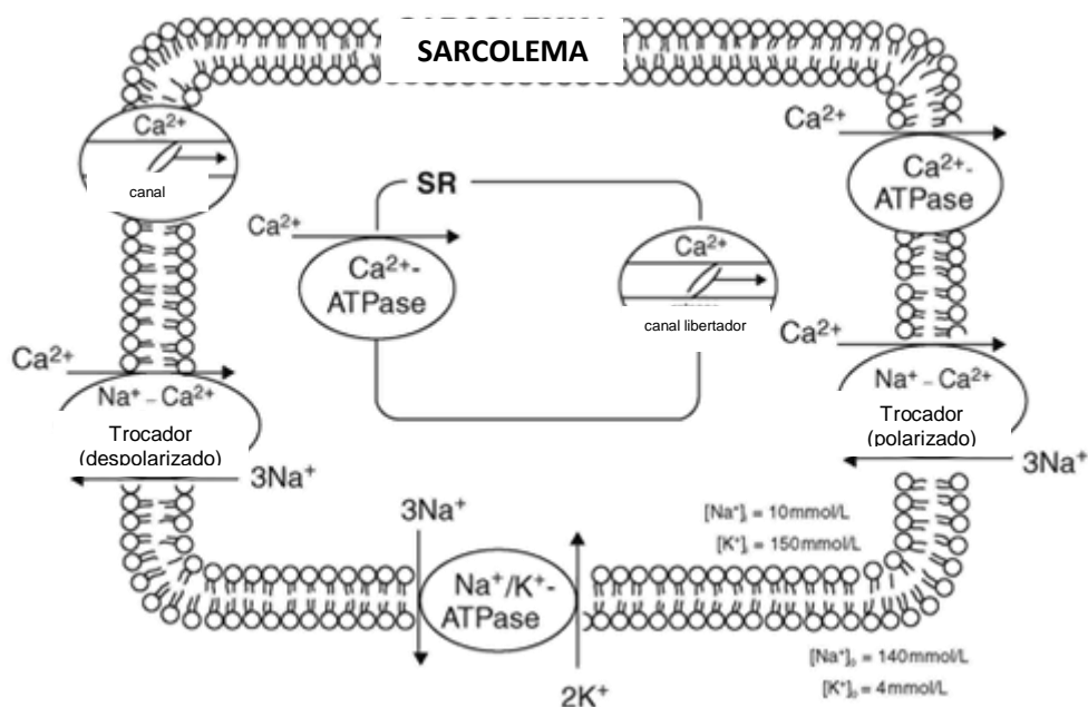
Figura 3.4: Mecanismo de ação da digoxina no sarcolema (adaptado de Lelie 44 )
