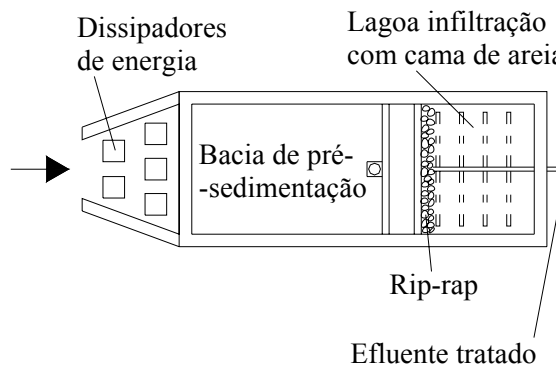
Fig. 7 – Filtros de areia. Fonte: Adaptado de Liu e Lipták (2000).
