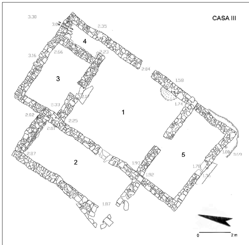
FIGURA 28. Planta geral da CASA III, SÍTIO 3.
