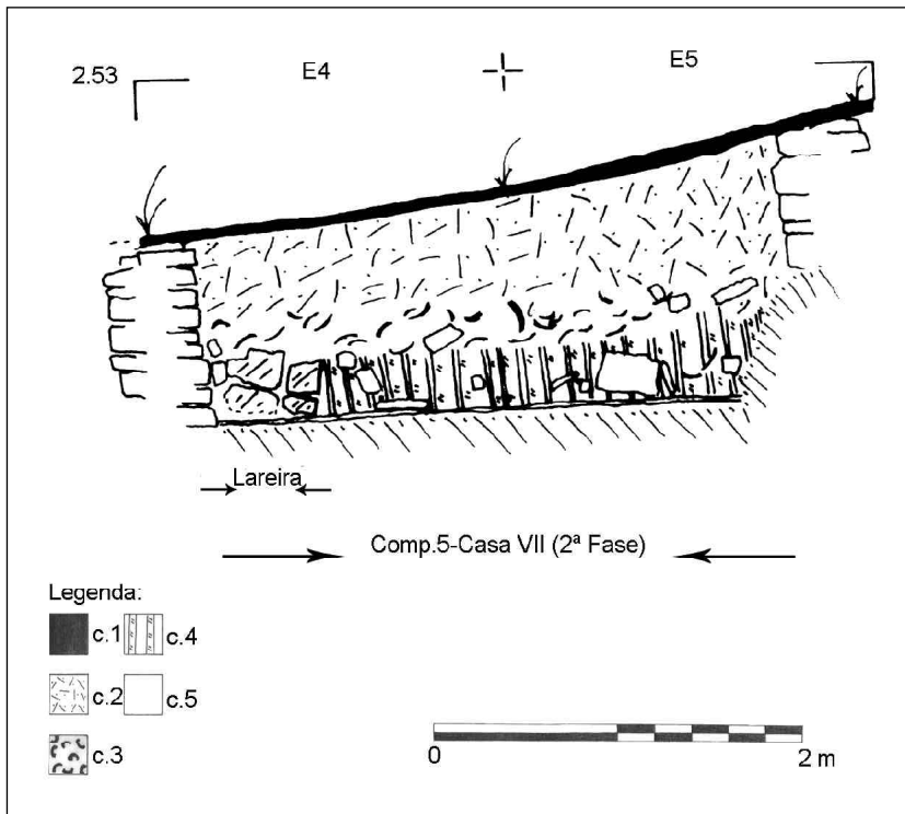
FIGURA 18. Corte estratigráfico 3 (E4-E5), SÍTIO 2, perfil noroeste/sudeste.
