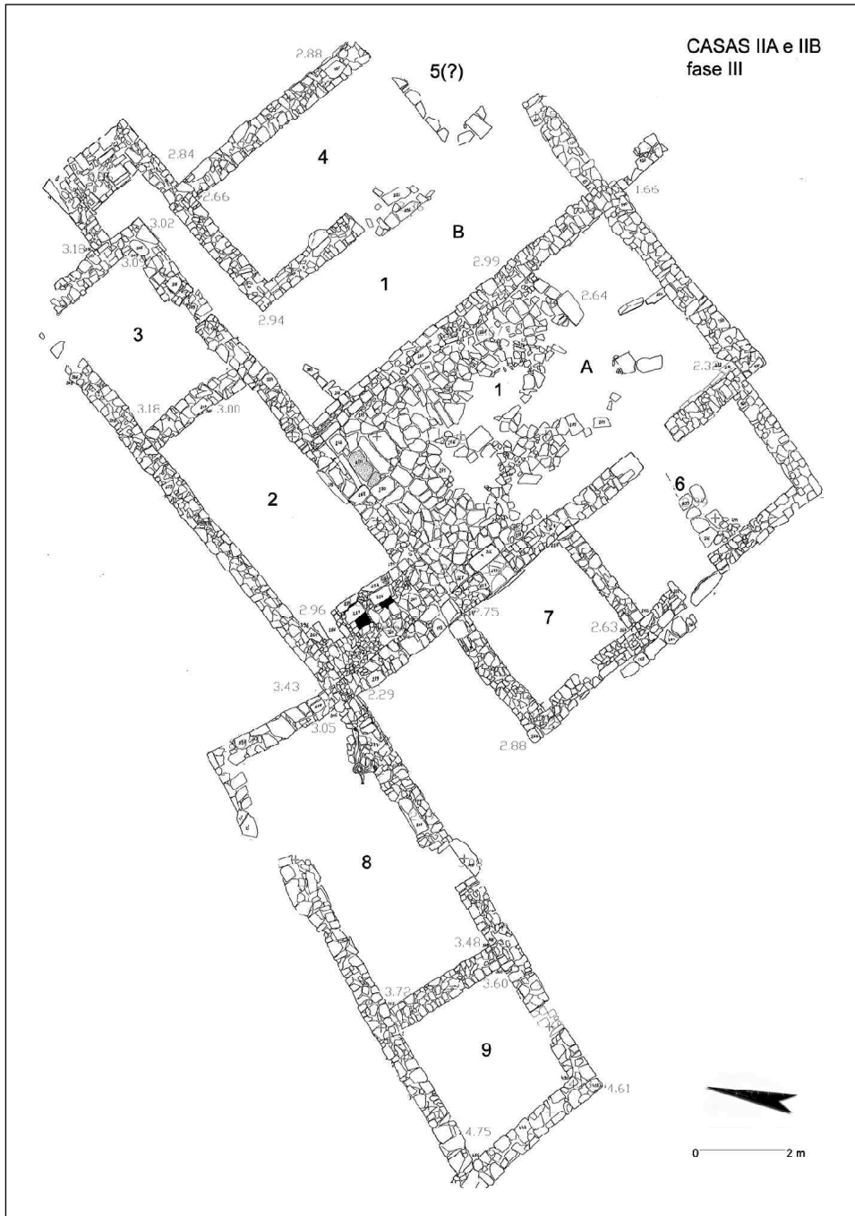
FIGURA 20. Planta geral da CASA IIA e IIB (fase III), SÍTIO 3.
