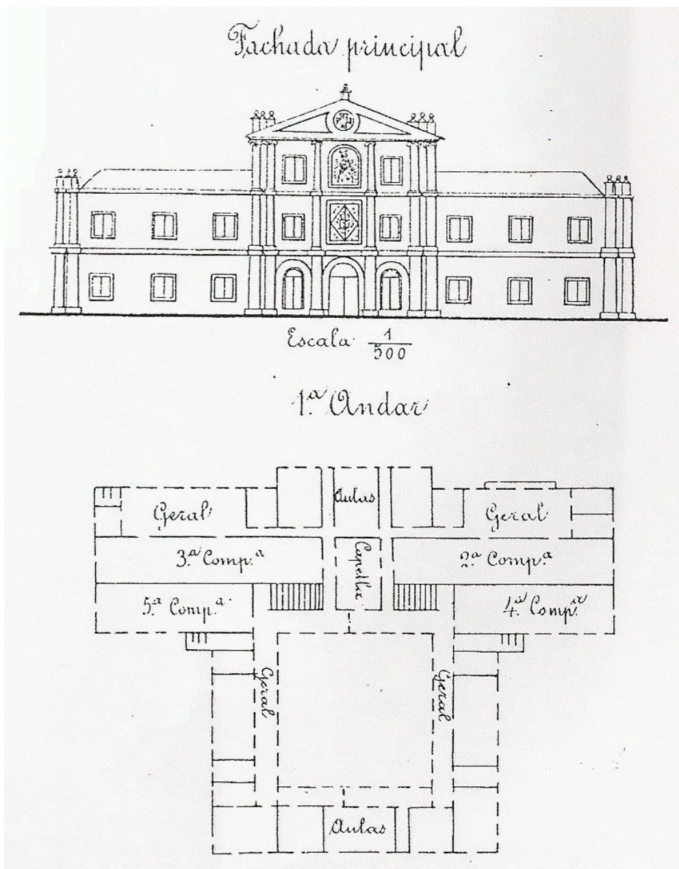
Ilustração 46: Alçado frontal e planta do 1º piso do antigo Hospital da Luz de Carnide no final do século XIX.
