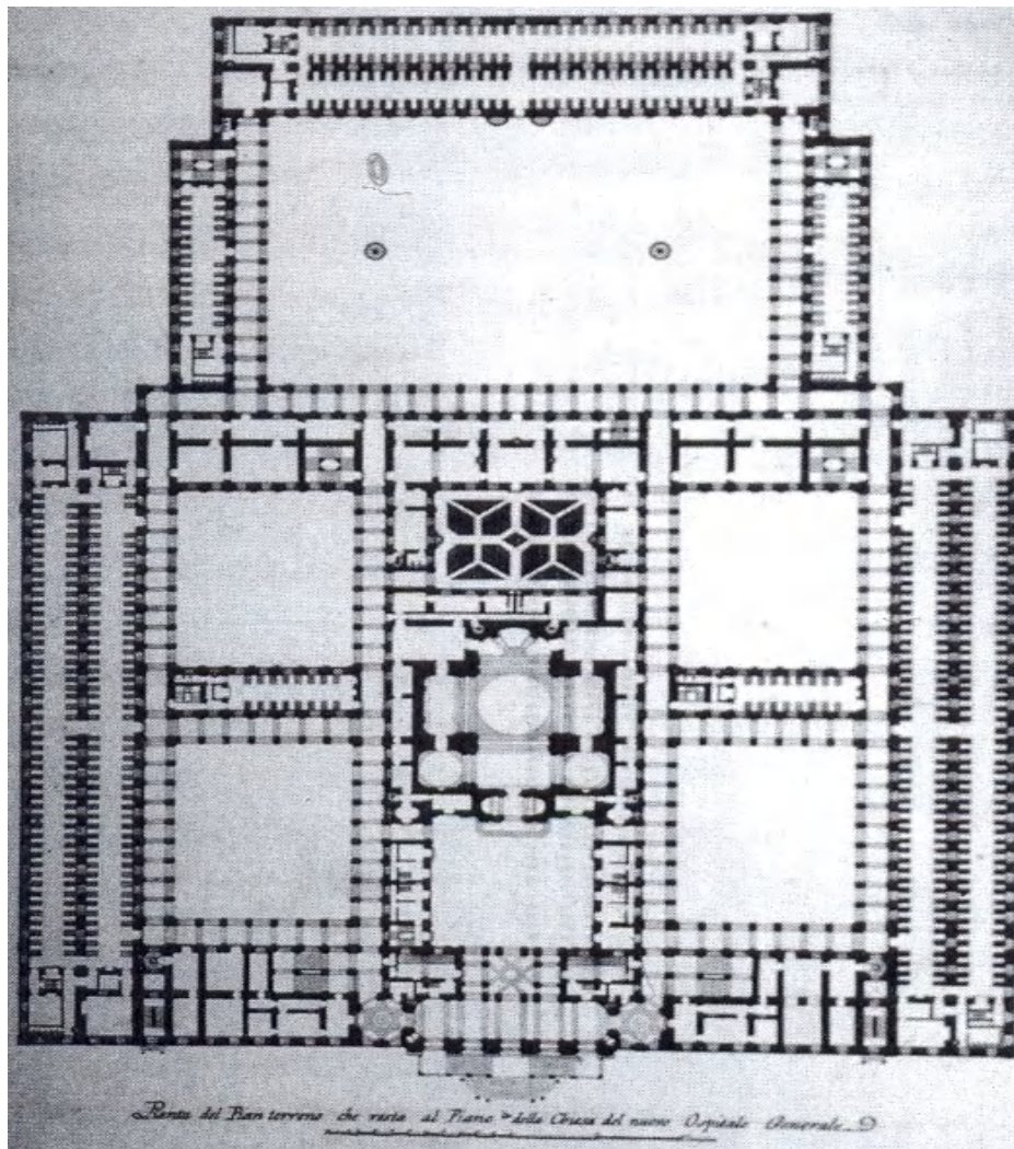
Ilustração 42: Planta do Hospital Geral de Madrid.
