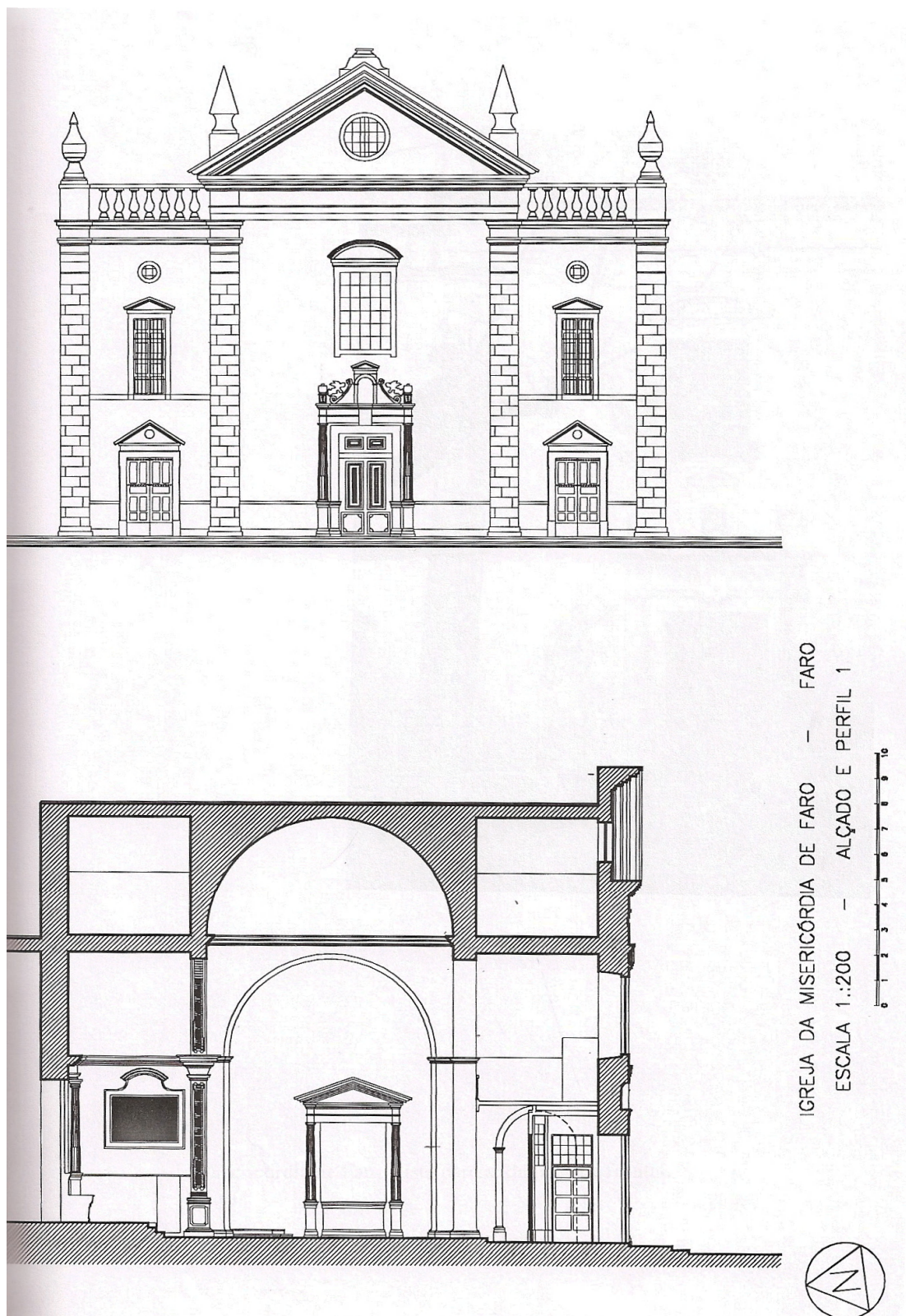
Ilustração 76: Alçado da Igreja da Misericórdia de Faro.
