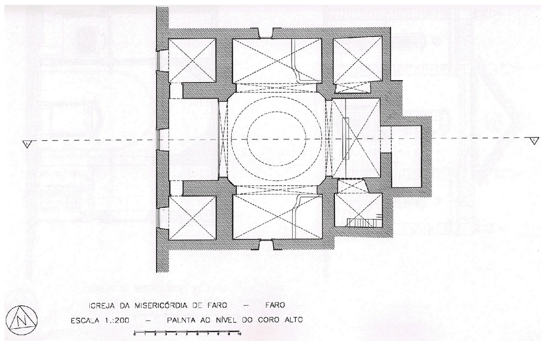
Ilustração 77: Planta da Igreja da Misericórdia de Faro.
