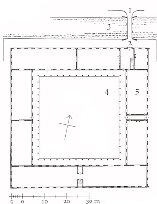
11. Leiden. Ehem. Pesthaus. Grundriß (vor Veränderungen des 19. Jh.), nach Inventar. 1 Brücke, 2 Portal, 3 Wassergraben, 4 Hof, 5 Krankensäle.
