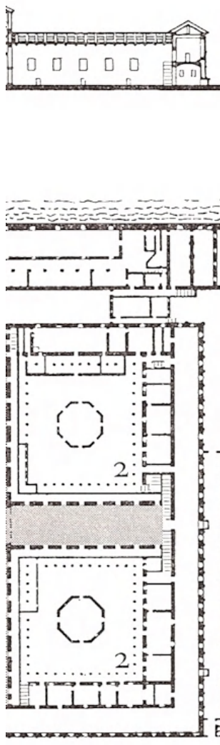
Ilustração 86: Parte da planta do Ospedale Maggiore de Milão apresentado acima no texto.
