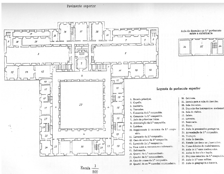
Ilustração 48: Planta do Antigo Hospital da Luz de Carnide.
