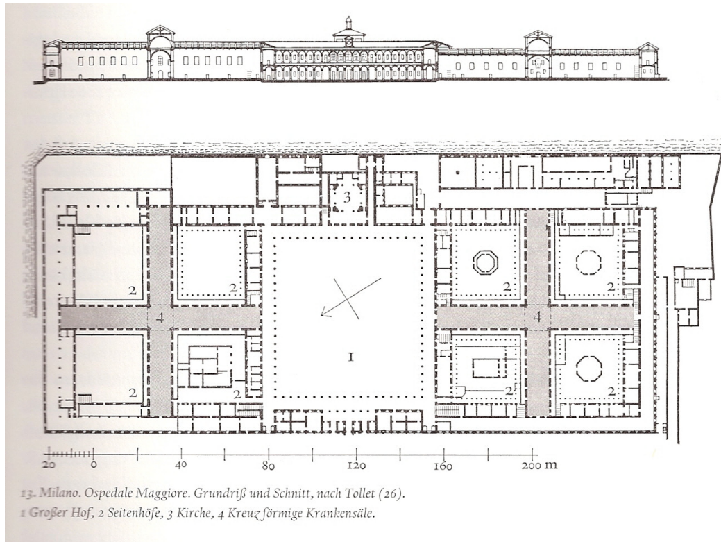
Ilustração 31: Planta do Ospedale Maggiore, Milão.
