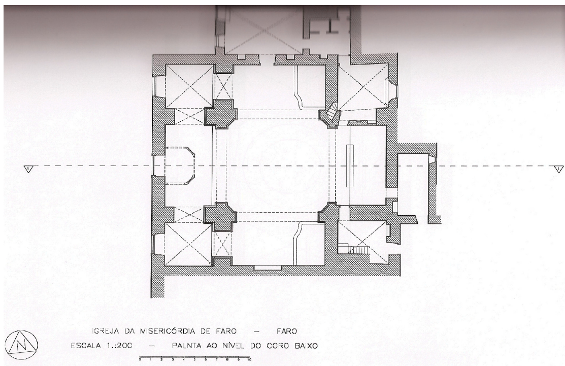
Ilustração 78: Planta da Igreja da Misericórdia de Faro.
