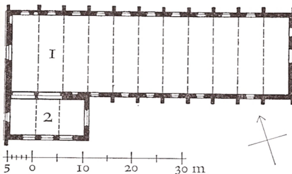
4. Gent. Hospital Biloke, Grundriß, nach van Puyvelde (33). 1 Hospitalhalle, 2 Kapelle.
