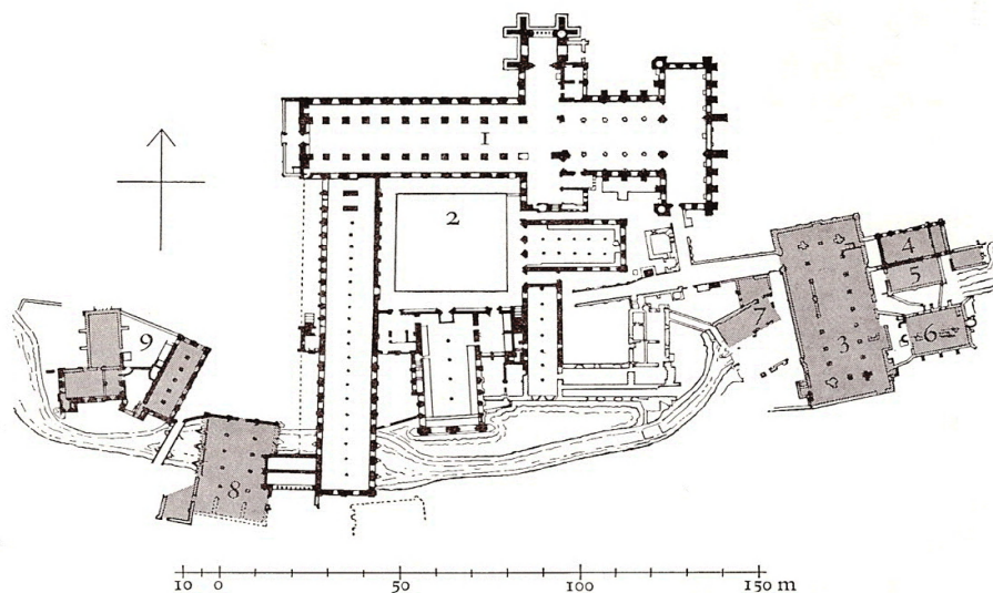
3. Fountains Abbey. Grundriß und Ansicht (Rekonstruktion), nach Fletcher (82). 1 Klosterkirche, 2 Klausur, 3 Infirmerie der Mönche, 4 Raum des Infirmarius (darunter Keller), 5 Kapelle, 6 Küche, 7 Misericord,
