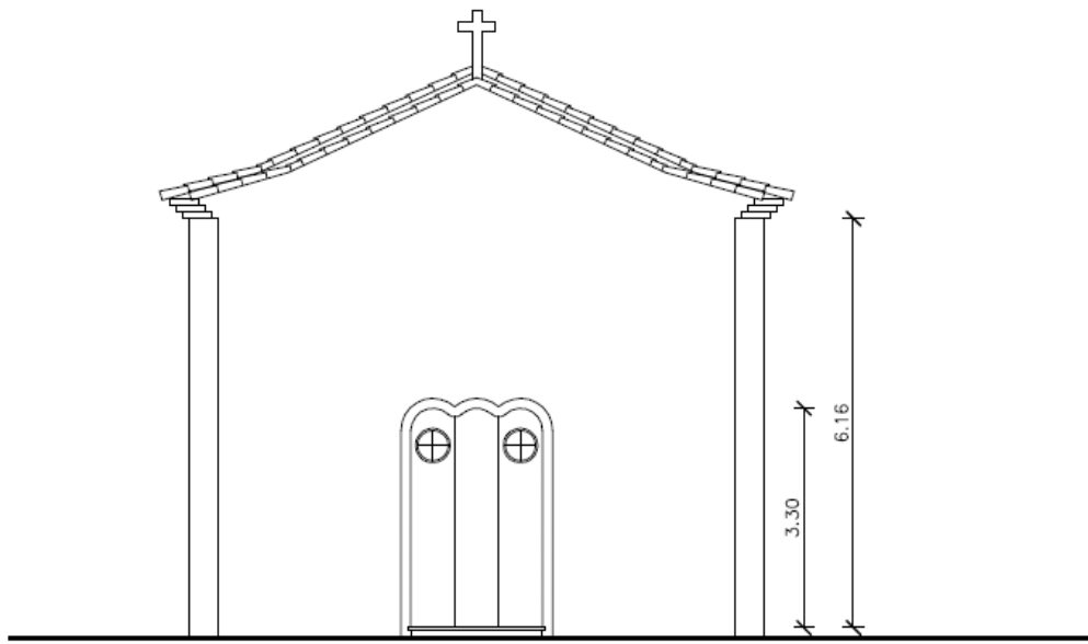
Ilustração 70: Idem; conjectura: vista 2.
