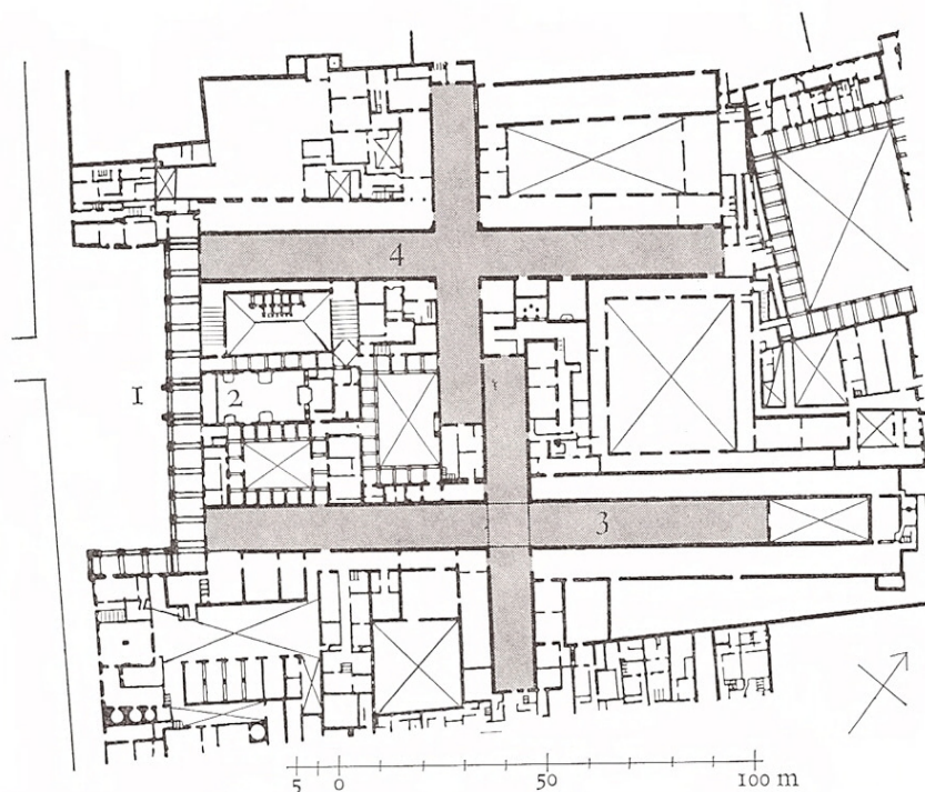
12. Firenze. Hospital S. Maria Nuova. Lageplan (Rekonstruktion), nach Paatz (22). 1 Zugang mit Loggia, 2 Kirche S. Egidio, 3 Männersaal, 4 Frauensaal.
