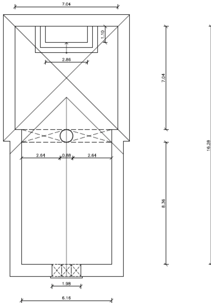
Ilustração 69: Planta da Ermida do Espírito Santo; conjectura: vista 1.
