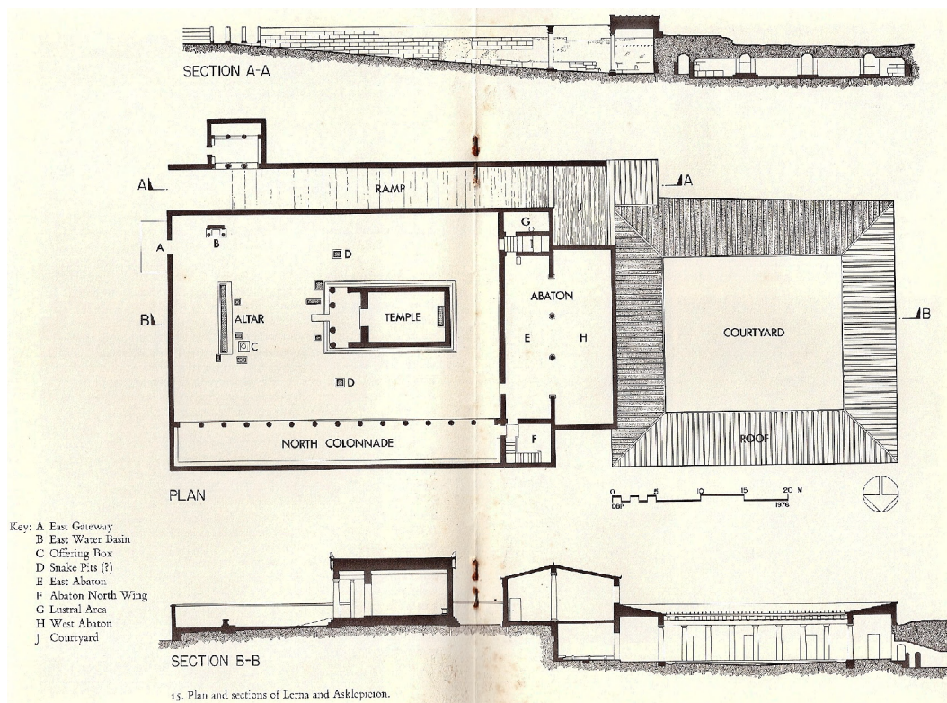
Ilustração 8: Planta de Lerna e Aesklepion de Corinto.
