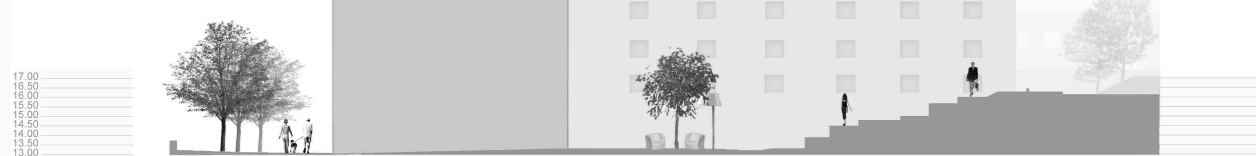
Perfil C-C'
