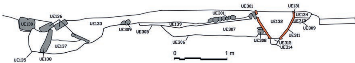
Figura 9 – Perfil estratigráfico W-E do lagar.
