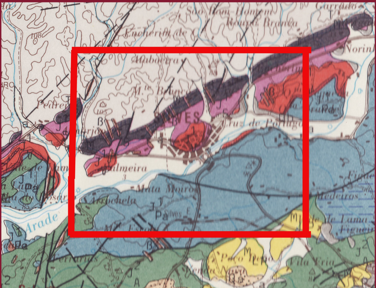
Carta Geológica do Algarve 1:100 000 - Folha Ocidental - Região de Silves
