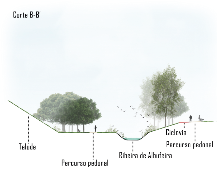
Cortes à escala 1/500
