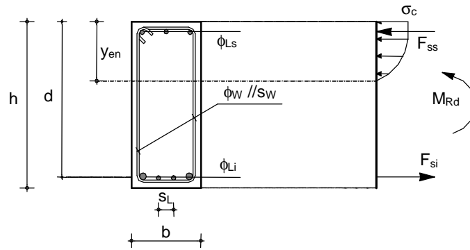
Figura 3: Secção de betão armado de largura “b” e altura “h” a otimizar.
